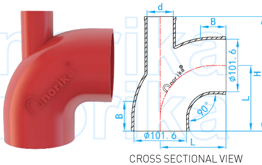
4"x2"x90 DEG BEND
